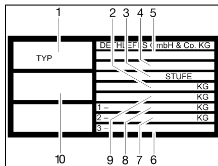
Bild 298 Typschild
