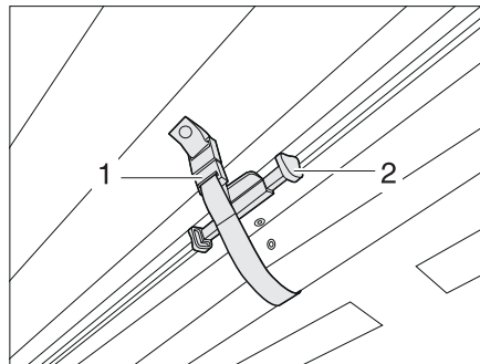
Bild 59 faltverdunklung für die Frontscheibe
