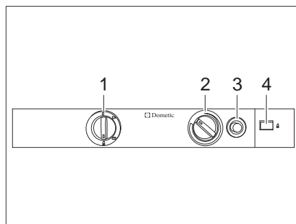
Bild 242 Bedienelemente für den Kühlschrank (Dometic 8er-Reihe)
