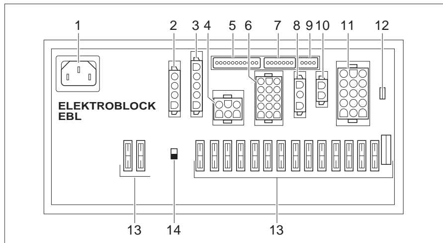
Bild 193 Elektroblock (EBL 102)
