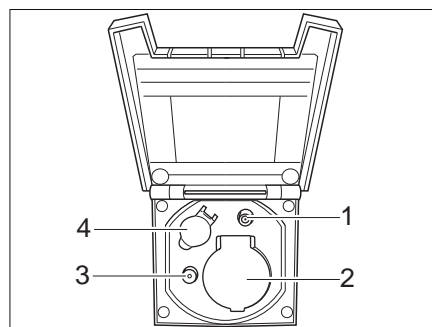
Bild 25 Kabelanschluss
