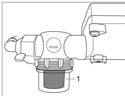
Bild 287 Wasserfilter der Druckwasserpumpe
