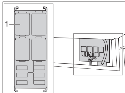
Bild 208 Fiat-Sicherungen im B-Holm unten auf der Beifahrerseite
