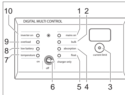
Bild 196 Panel IT 992
