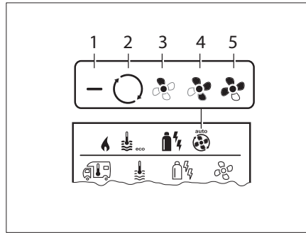
Bild 203 Einstellmöglichkeiten Gebläse Heizung
