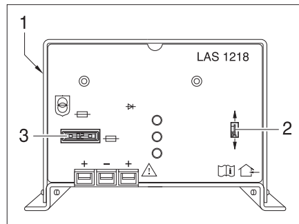
Bild 191 Zusatz-Ladegerät
