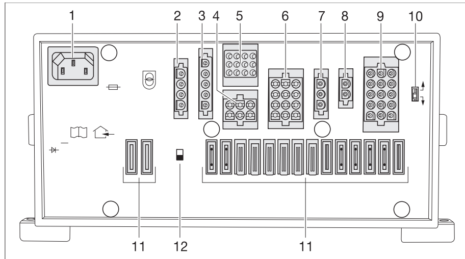
Bild 192 Elektroblock (EBL 99)
