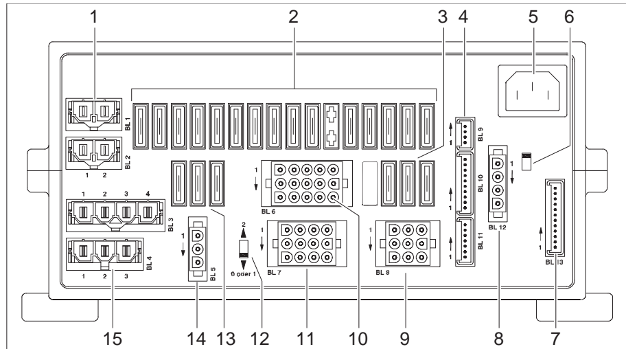
Bild 194 Elektroblock (EBL 220)
