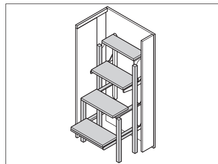
Bild 41 4-stufige Leiter
