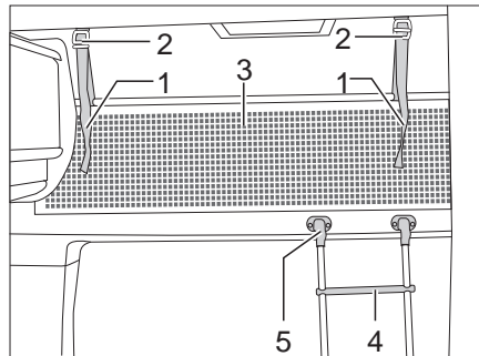
Bild 110 Alkovenbett
