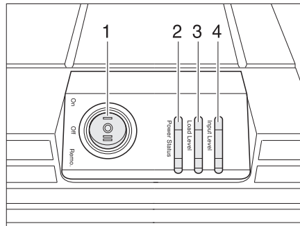
Bild 189 Anzeigen und Bedienelemente
