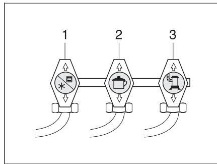
Bild 180 Symbole der Gasabsperrventile alternativ
