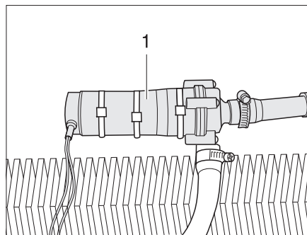
Bild 219 Zusatz-Umwälzpumpe
