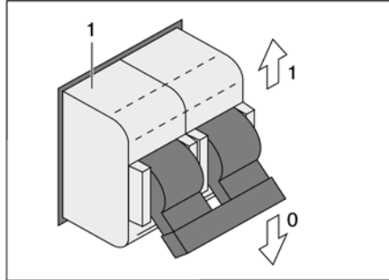
Bild 212 230-V-Sicherungsautomat
