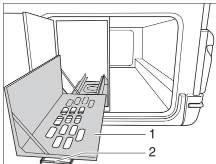
Bild 177 Gaskasten, mit ausziehbarem Schlitten (Variante 2)
