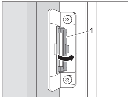
Bild 254 Arretierung in Ausgangslage zurück drehen
